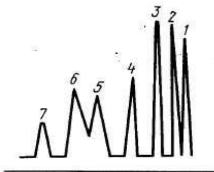
Рис.17. Хроматограммы смеси воды и кислот (115° С):
