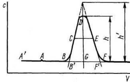
Рис.15. Кривая проявительного анализа (хроматографический пик)
