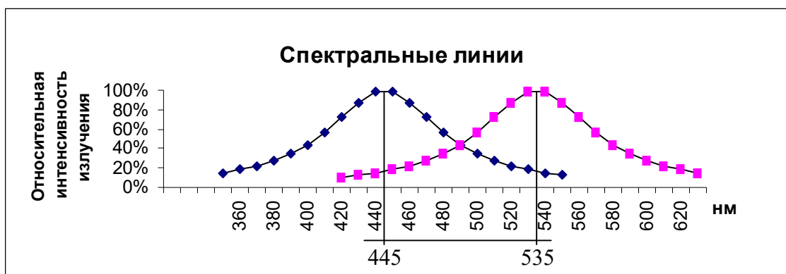
Рис. 11. Стоксово смещение
