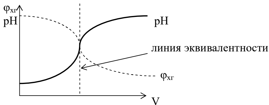
Рис.4. Кривая потенциометрического титрования
