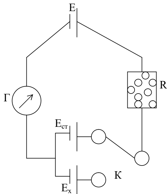
Рис.2. Компенсационная схема
